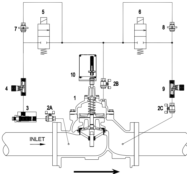
Schematic A-7637A
